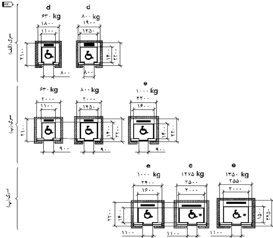
شکل ۵ آسانسورها با کاربرد عمومی
