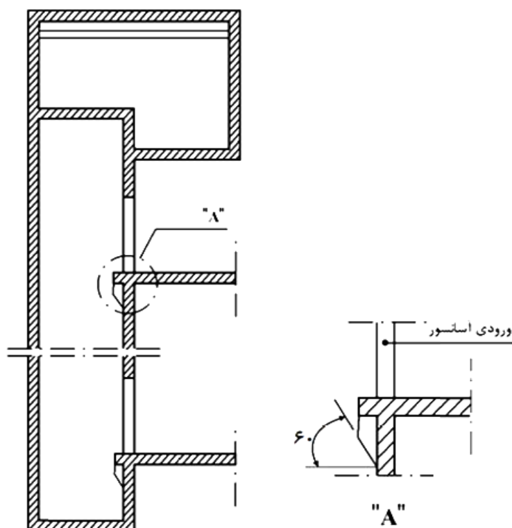
شکل ۱۵-۲-۲-۳ سطح داخلی دیواره چاه در سمت ورودی طبقات.
