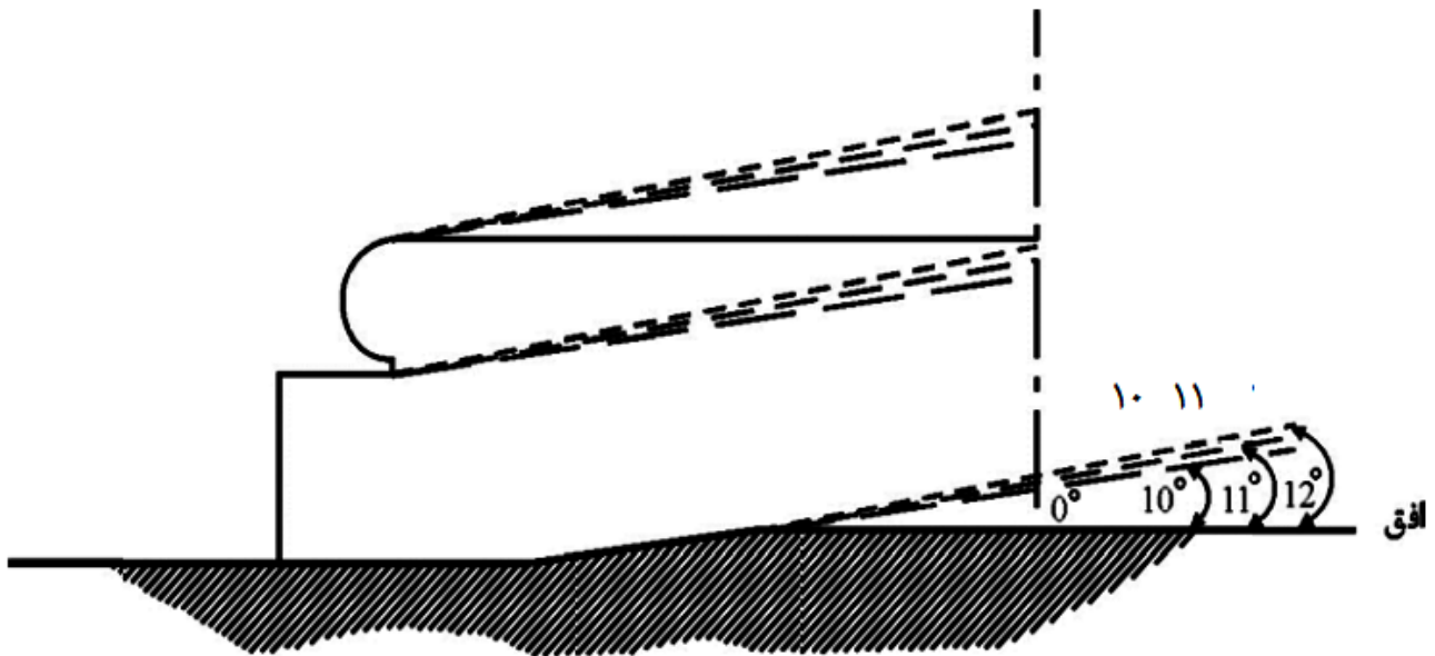
شکل ۱۵-۳-۱۲ زوایای شیب پیاده‌روهای متحرک
