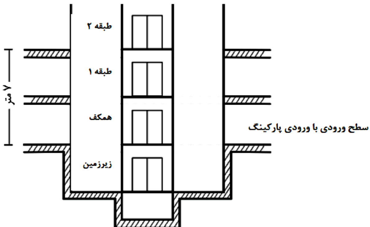
شکل ۱ روش تعیین حداکثر ارتفاع در ساختمانهای مسکونی
