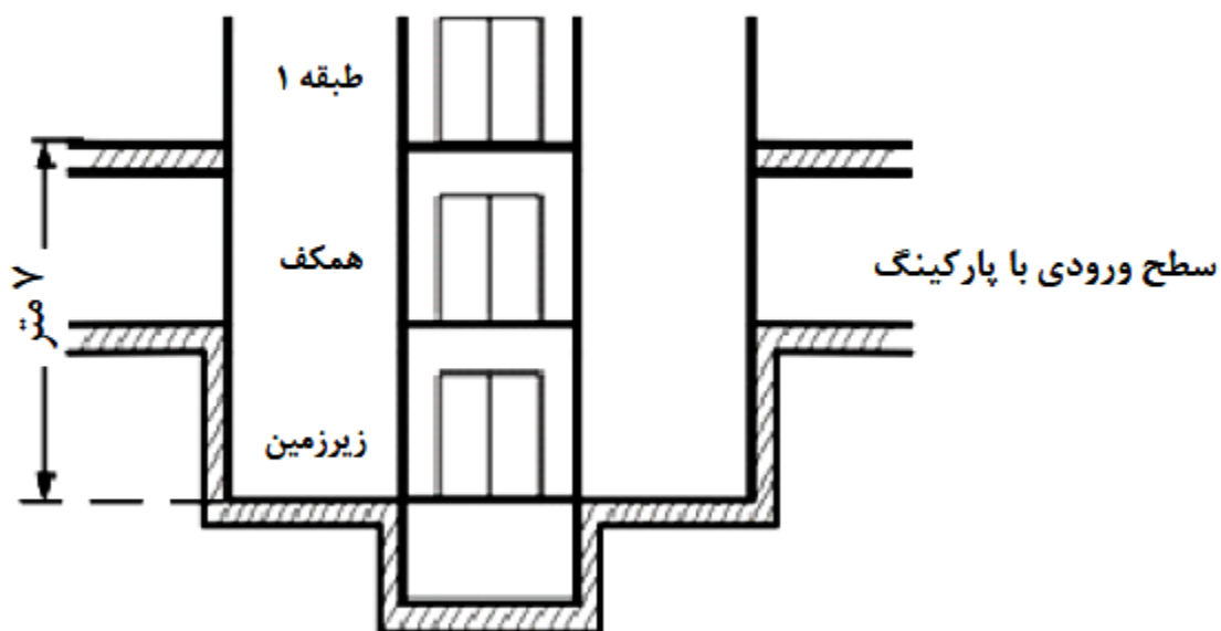
شکل ۲ روش تعیین حداکثر ارتفاع در ساختمانهای غیرمسکونی
