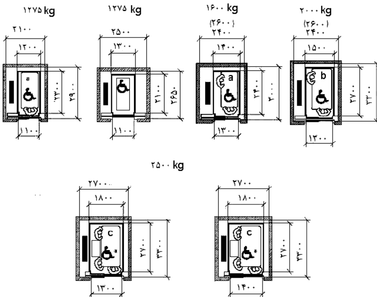
شکل ۷ آسانسورهای بیمارستانی
