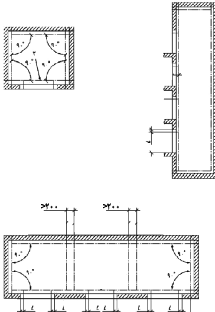
شکل ۱۵-۲-۲-۹-۳ خطوط شاقولی و دیواره‌های جداساز چاه‌های آسانسور
