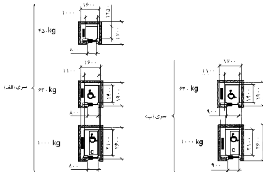
شکل ۴ آسانسورهای ساختمان مسکونی
