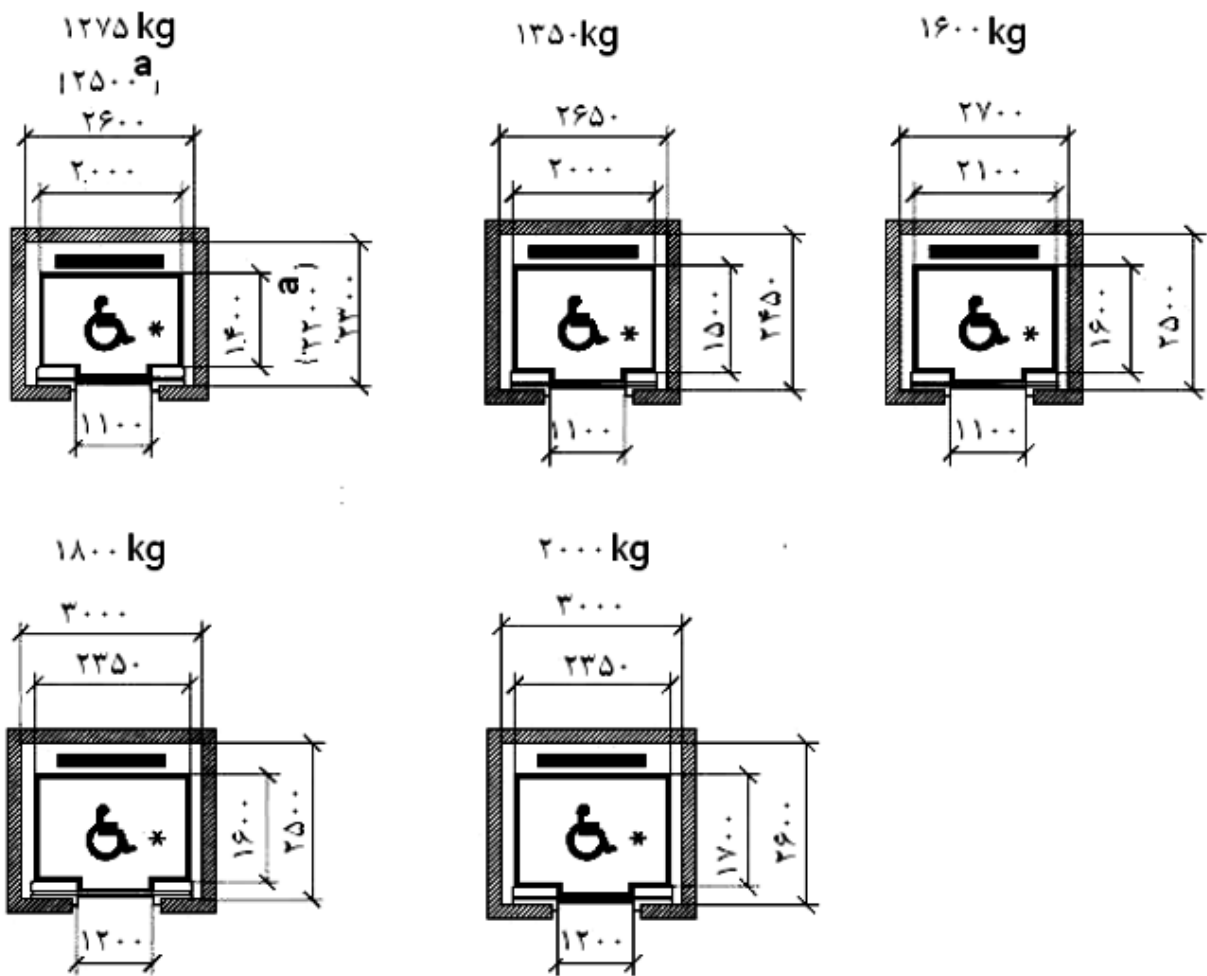
شکل ۶ آسانسورهای با ترافیک سنگین
