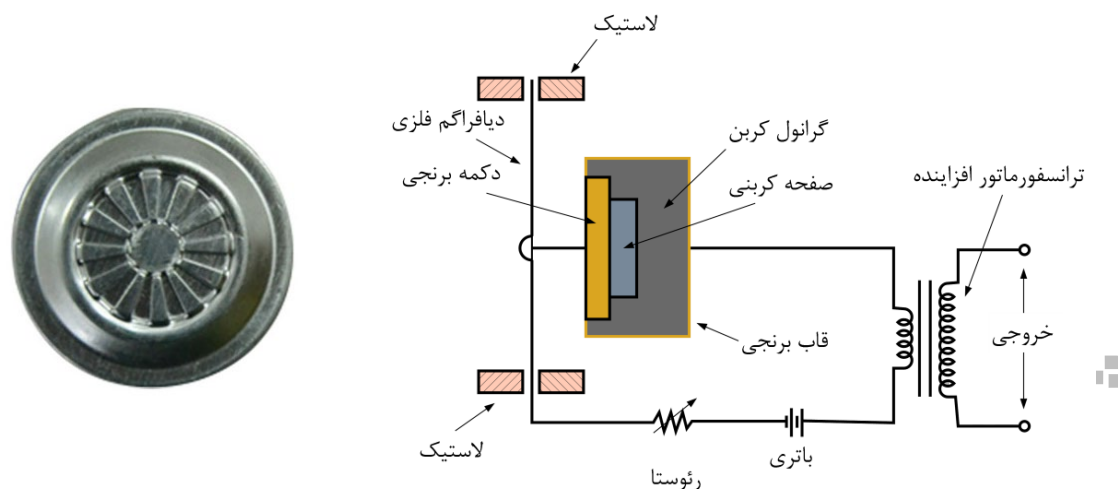
شکل ۷-۲۹- ساختمان داخلی و یک نمونه کپسول میکروفن کربنی
