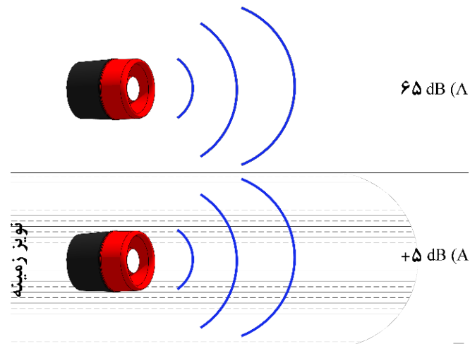
شکل ۴-۲۰- تاثیر نویز زمینه در طراحی شدت صوت آذیر
