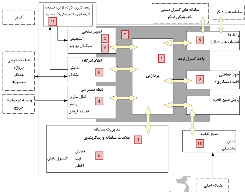
شکل ۳-۳۰- معماری عمومی سیستم کنترل دسترسی الکترونیکی
