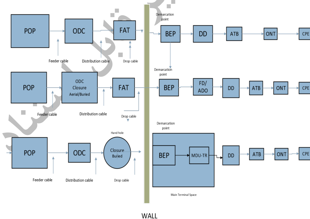
شکل ۱-۱۶- نمونه‌هایی از اصطلاحات طراحی شبکه فیبر نوری ساختمان‌ها در ایران
