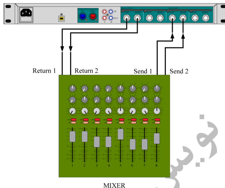
شکل ۶۷-۷- بلوک دیاگرام اتصال افکت پروسسور به میکسر صوتی
