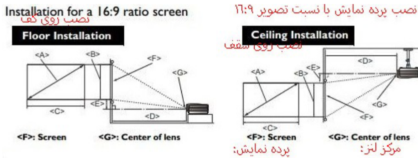
شکل ۸-۳۳ - یک نمونه ابعاد مختلف پرده و فاصله ویدیو پروژکتور
