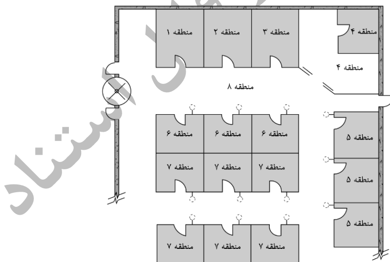
شکل ۴-۱۸- الف- نمونه تخصیص منطقه کشف برای مناطق مجاور و غیر همجوار
