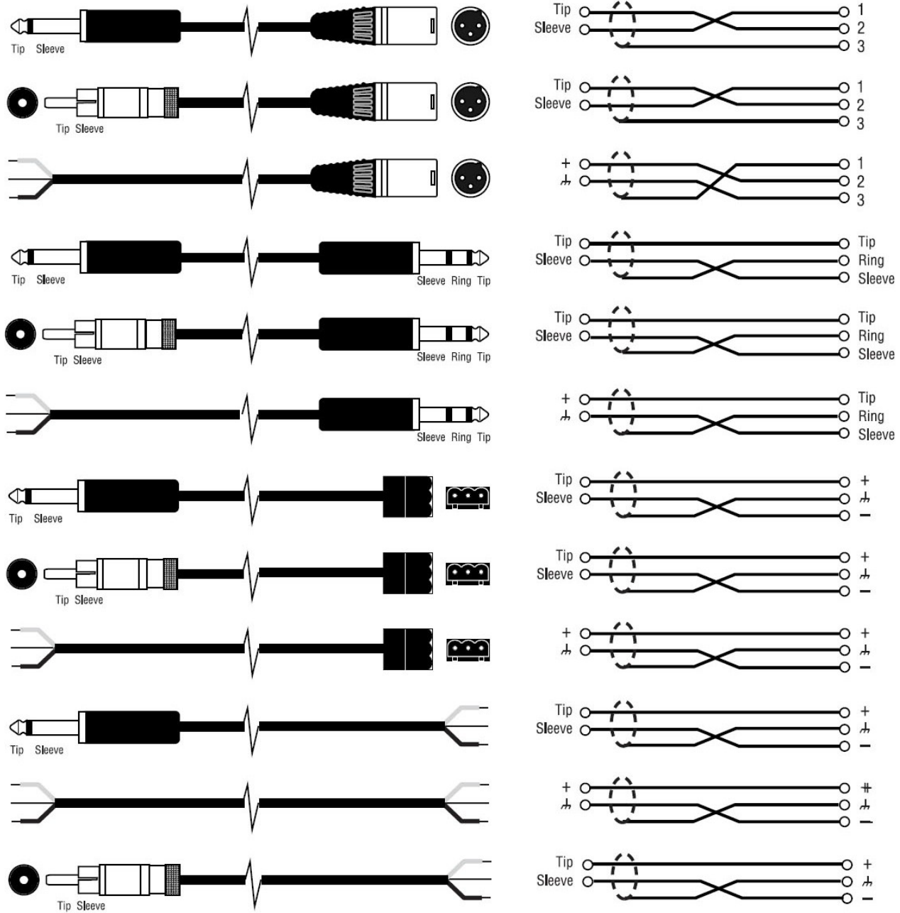
شکل ۷-۱۵۸- نحوه اتصال خروجی سیگنال نامتوازن به ورودی متوازن با اتصالات مختلف
