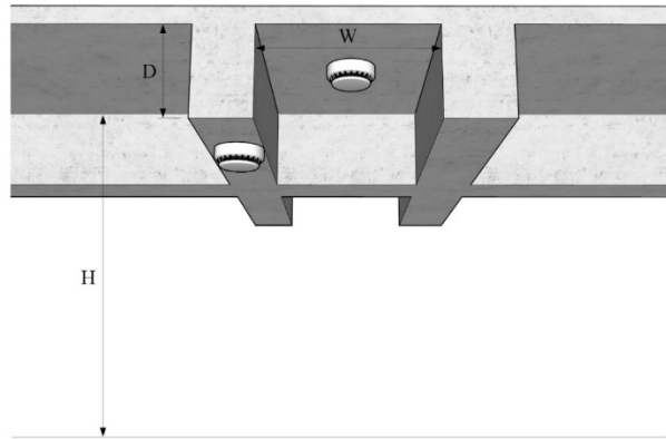
شکل ۴-۴۵- سقف افقی شامل سلول‌های کوچک
