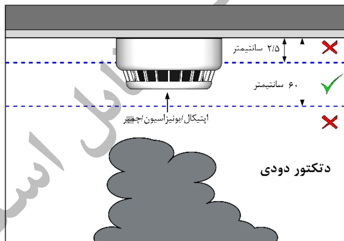
شکل ۴-۳۸- محدوده مجاز دتکتور دودی
