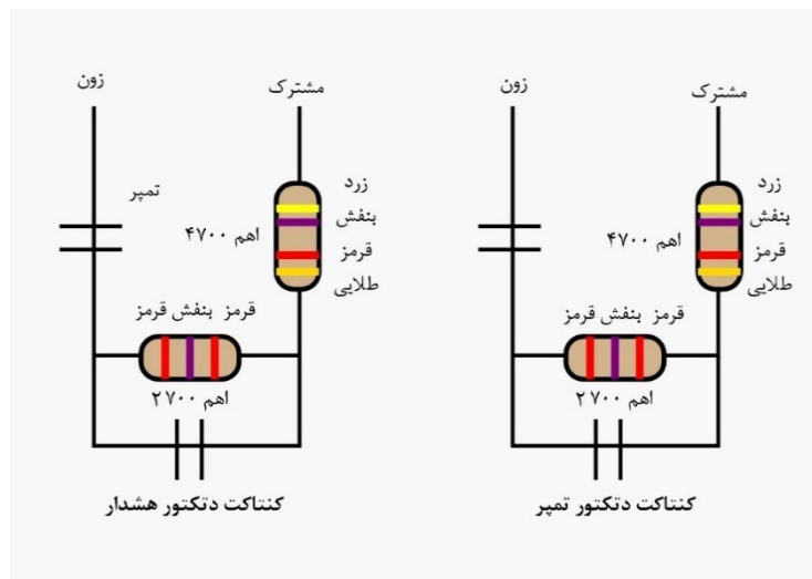
شکل ۳-۷- نحوه ارتباط دتکتورها با مرکز کنترل سیستم هشدار در درجه امنیت سه
