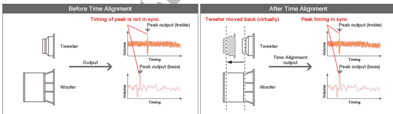
شکل ۴-۷ - ساختار و صدای خروجی دو بلندگو با واحد راه‌اندازهای با فاصله و واحد راه‌اندازهای هم تراز
