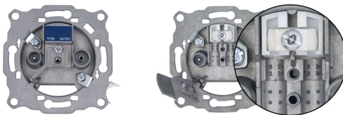
شکل ۲-۱۹- یک نمونه پریز میانی
