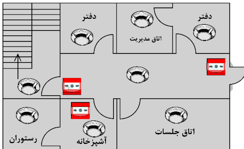
شکل ۴-۱۴- سیستم رسته حفاظت از جان
