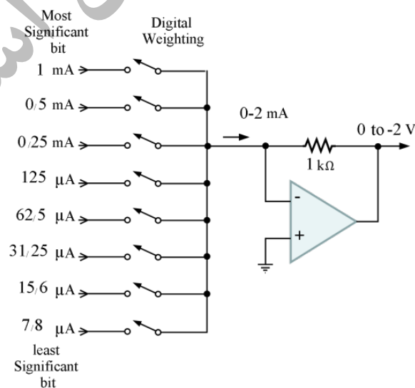
شکل ۷-۱۵- نمونه ساده‌شده مبدل متعارف نردبانی
