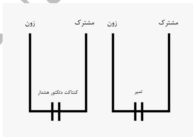
شکل ۳-۶- نحوه ارتباط دتکتورها با مرکز کنترل سیستم هشدار در درجه امنیت دو
