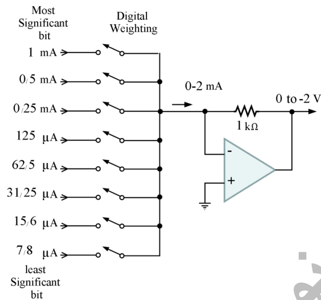
شکل ۷-۱۲- بلوک دیاگرام مبدل آنالوگ به دیجیتال فلش
