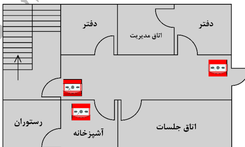
شکل ۴-۱۳- سیستم رسته دستی
