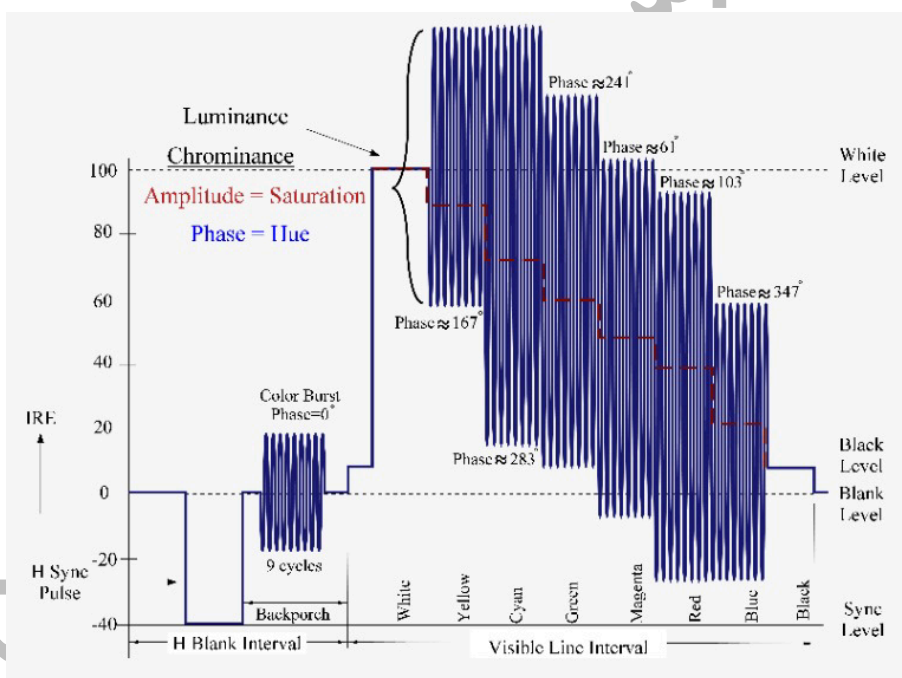
شکل ۸-۱۷- نمونه شکل موج سیگنال ویدیو رنگی
