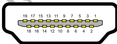
شکل ۲۸-۸- شماره پایه‌های کانکتورهای HDMI
