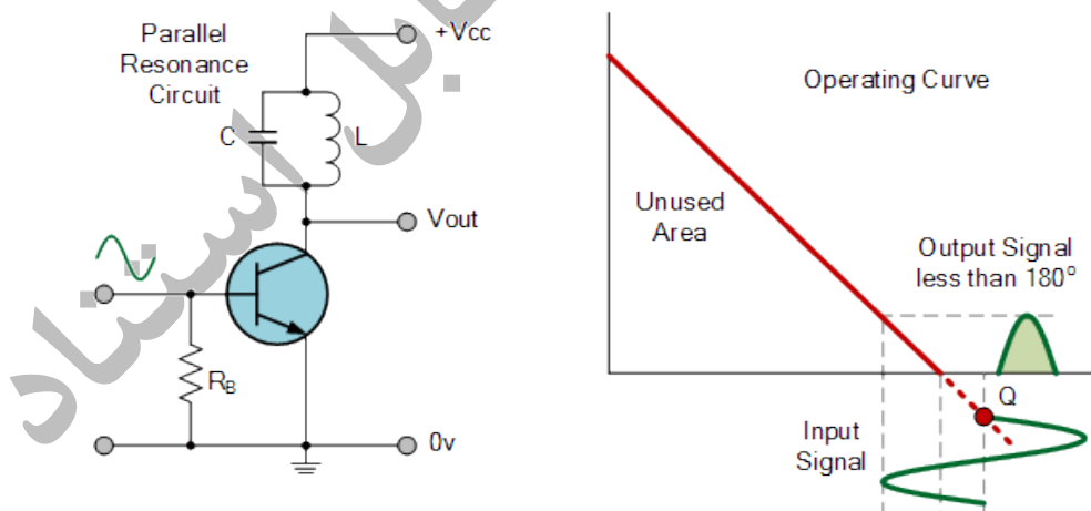
شکل ۷-۹۳- یک نمونه مدار ساده و منحنی نقطه کار و خط بار تقویت کننده کلاس C
