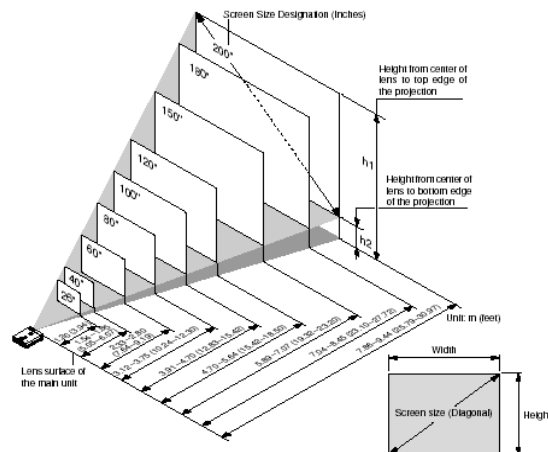
شکل ۸-۳۴ - یک نمونه فاصله ویدیو پروژکتور متناسب با ابعاد پرده
