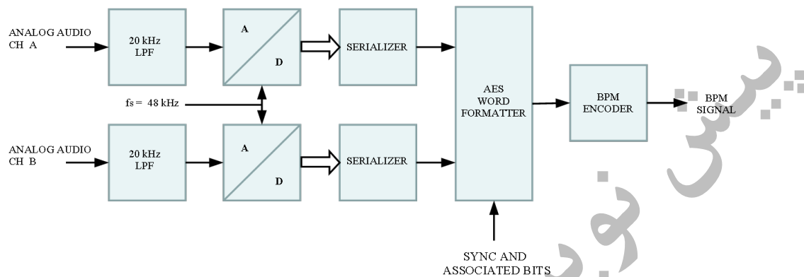
شکل ۷-۱۸- بلوک دیاگرام انکودر سیگنال دیجیتال AES/EBU
