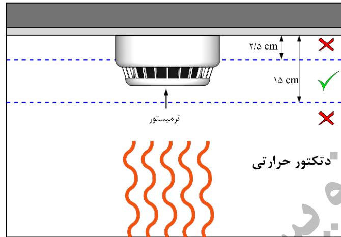
شکل ۴-۳۷- محدود مجاز جانمایی دتکتور حرارتی
