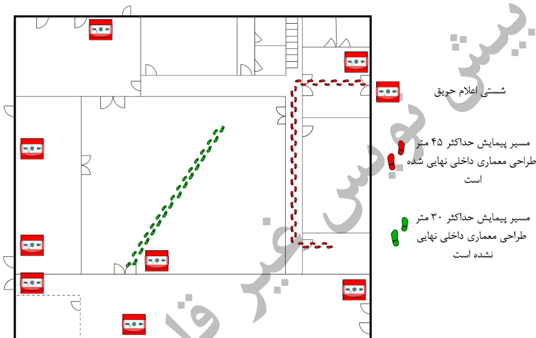
شکل ۴-۲۷- حداکثر پیمایش جهت فعال‌سازی شستی اعلام حریق
