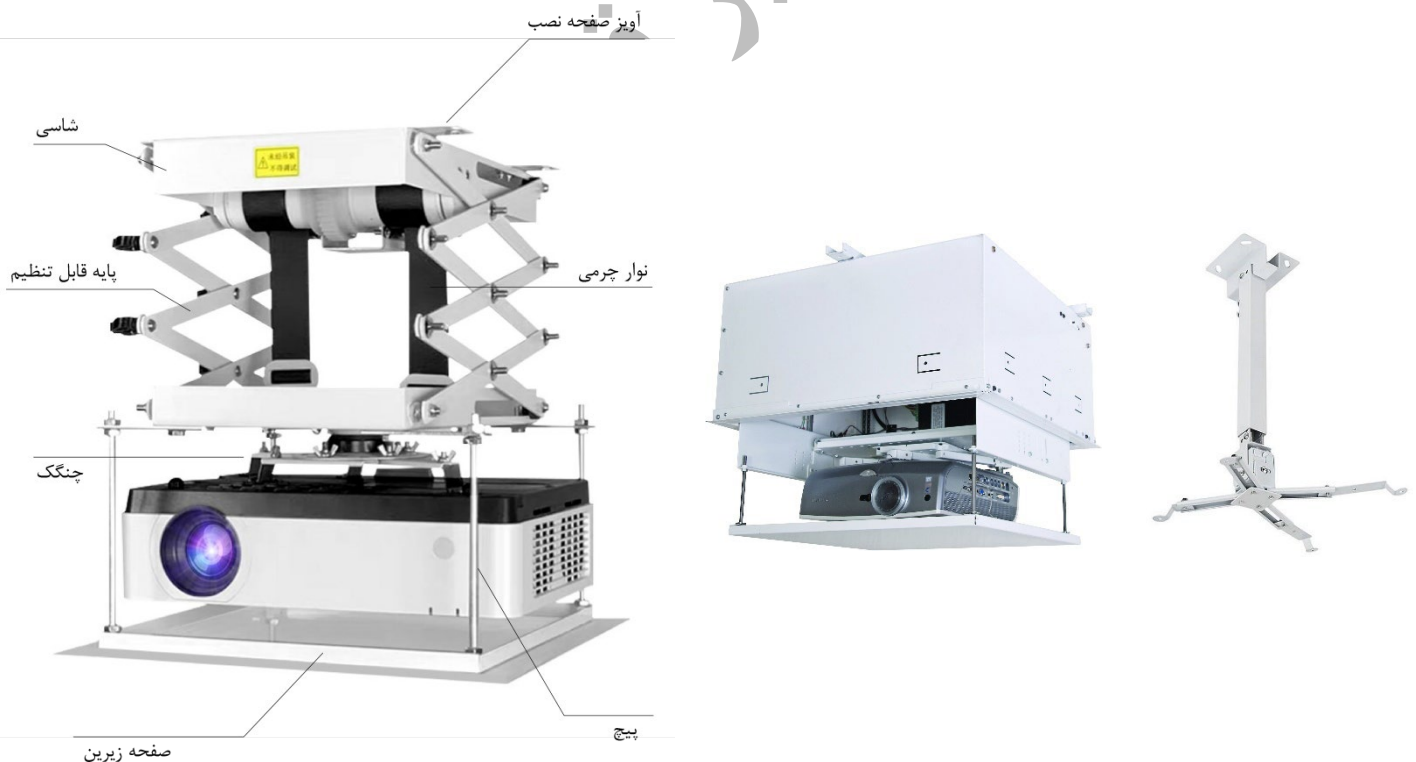
دو نمونه پایه ویدیو پروژکتور متحرک برقی
