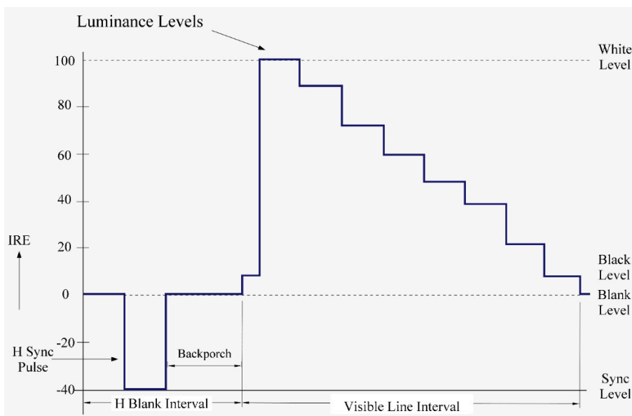
شکل ۸-۱۶- نمونه منحنی سیگنال تصویر سیاه و سفید
