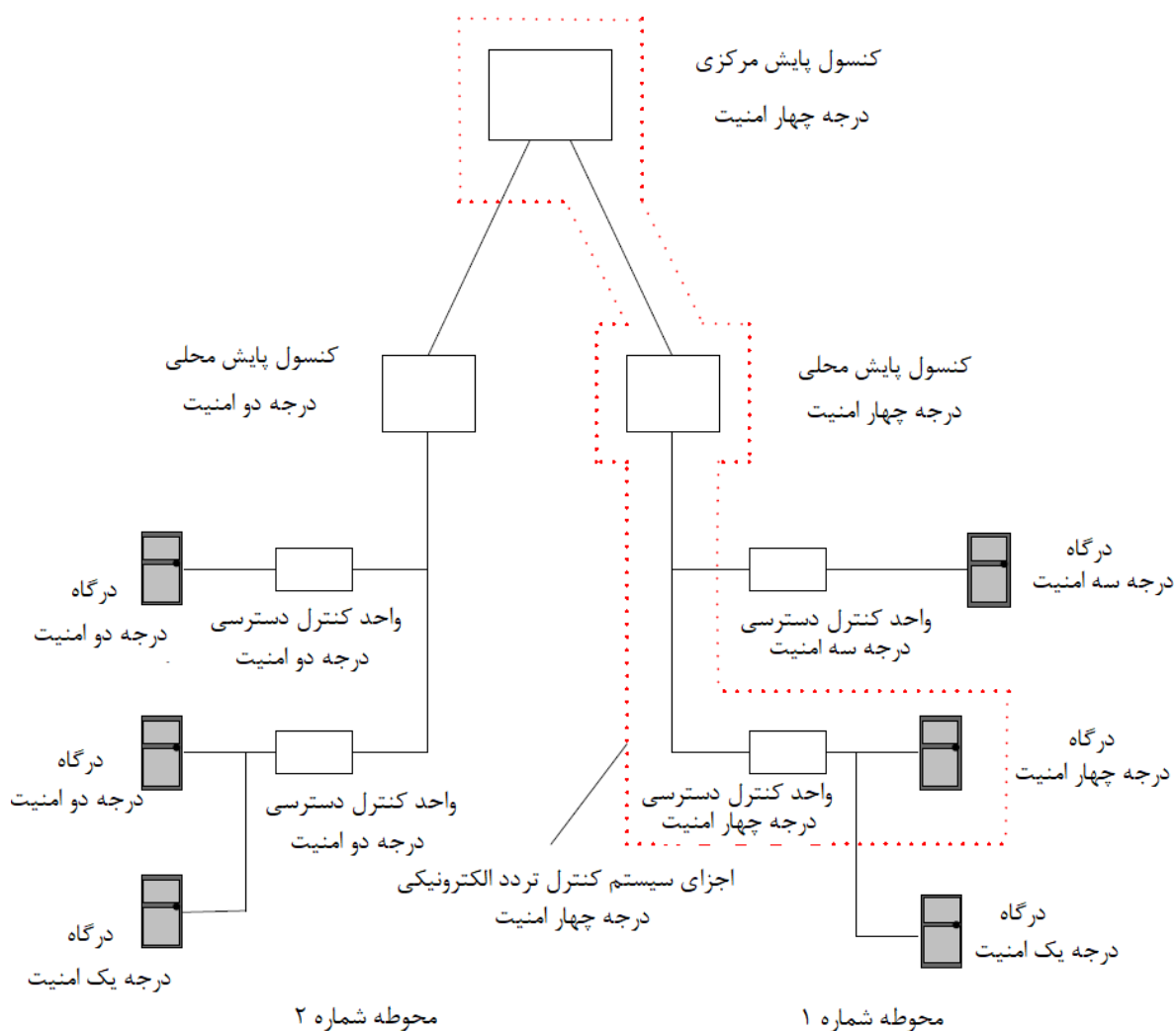
شکل ۳-۲۸- مثالی از انتخاب درجه امنیت در سیستم کنترل دسترسی الکترونیکی
