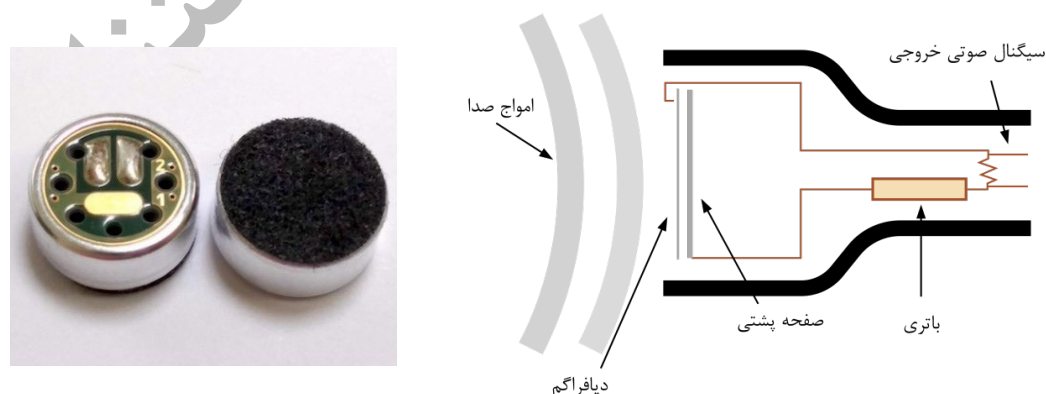
شکل ۷-۲۷- ساختمان داخلی و یک نمونه کپسول میکروفن خازنی
