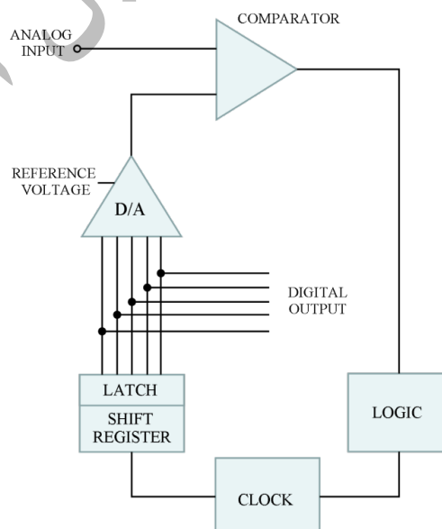
شکل ۷-۱۳- بلوک دیاگرام مبدل آنالوگ به دیجیتال تقریب متوالی
