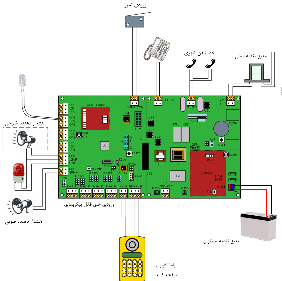
شکل ۳-۲- شمایی از یک مرکز کنترل سیستم هشدار
