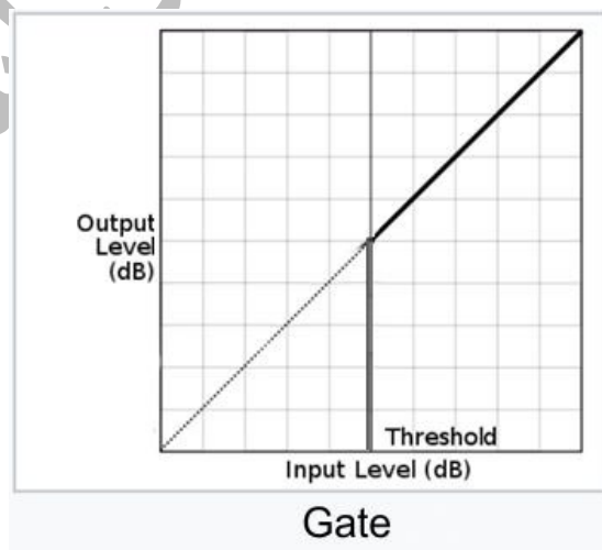
شکل ۷-۵۴- منحنی تابع دستگاه گیت
