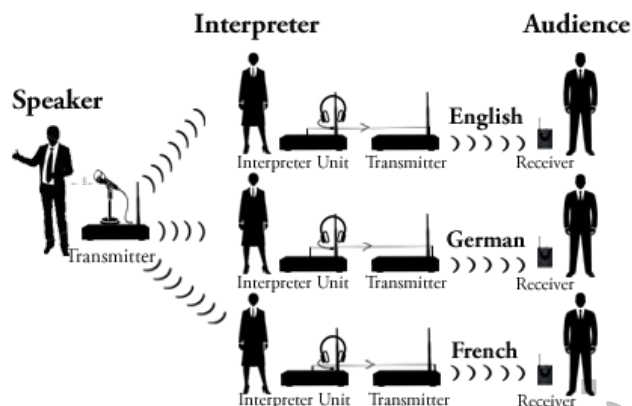
شکل ۸-۶- بلوک دیاگرام یک نمونه سیستم ترجمه هم‌زمان سه زبانه
