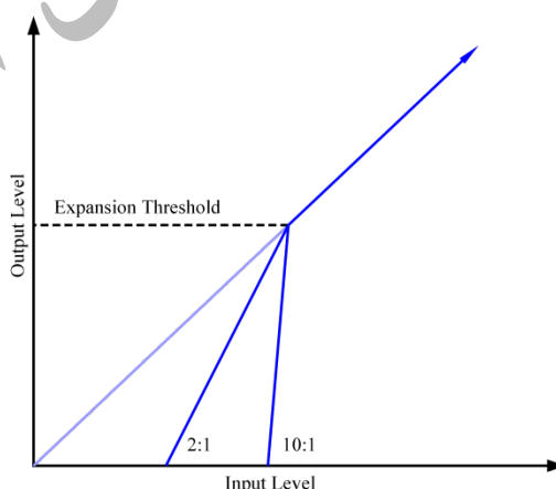
شکل ۷-۵۱- منحنی تابع دستگاه کمپرسور
