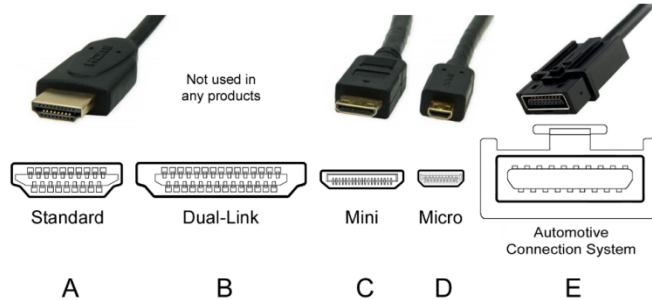
شکل ۲۷-۸- انواع مختلف کانکتورهای HDMI
