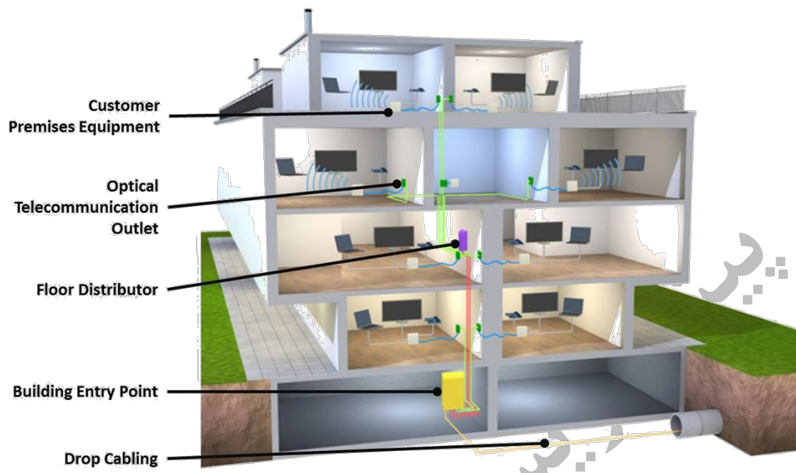
شکل ۱-۱۵- شماتیک ارتباطات نوری و تجهیزات ورودی و داخل ساختمان
