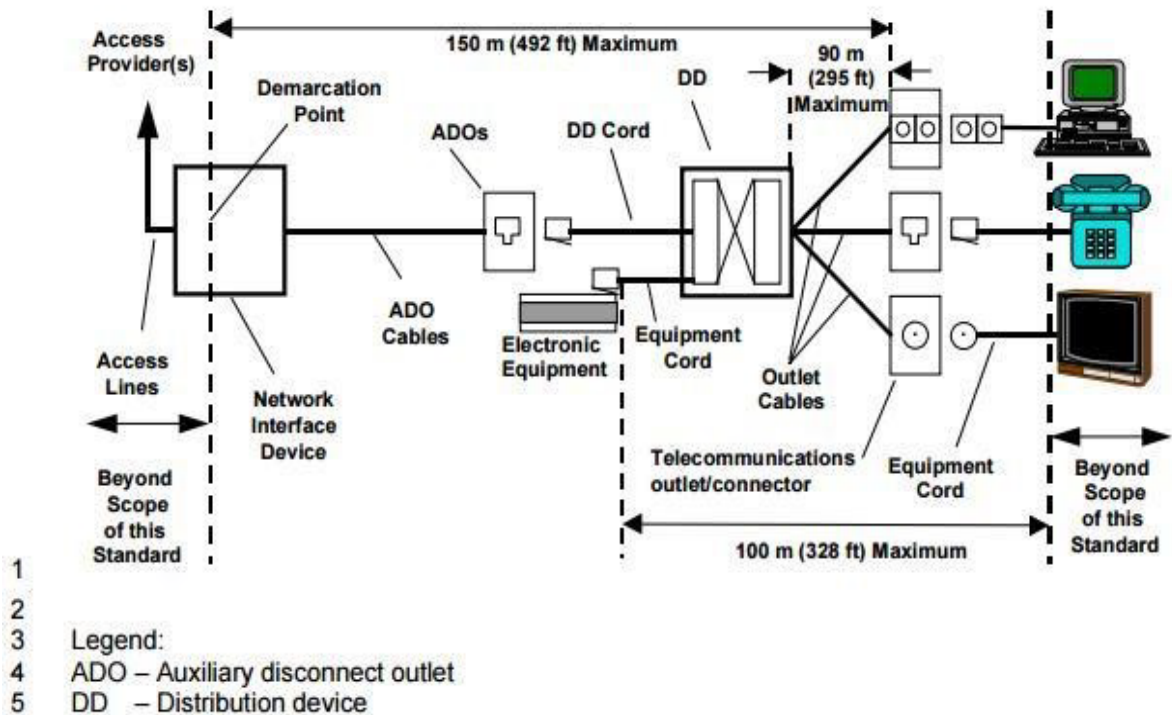
شکل ۱-۱۷- اجزای کابل کشی در یک واحد آپارتمان دوبلکس
