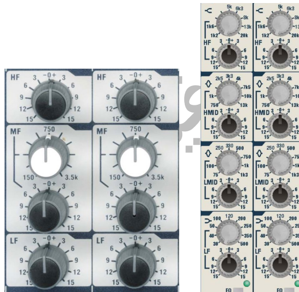
شکل ۷-۷ - دو نمونه پارامتریک اکولایزر
