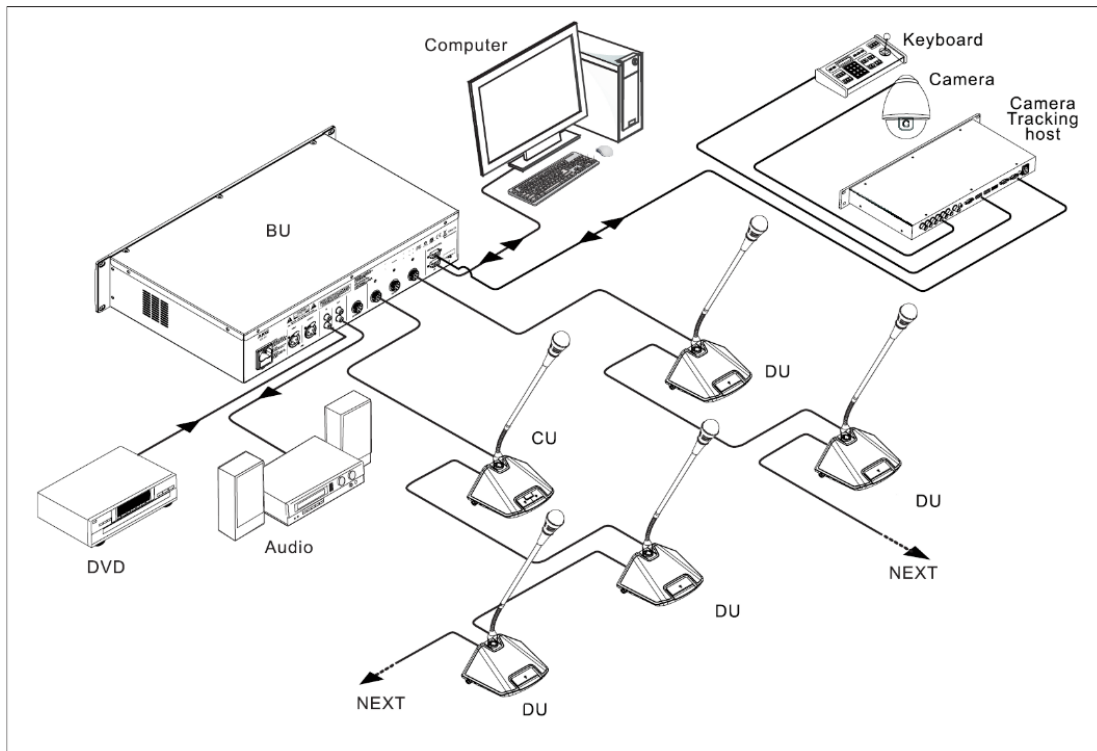
شکل ۸-۴۲- بلوک دیاگرام و اتصالات اجزاء یک سیستم کنفرانسی با تجهیزات دنبال‌کننده تصویری
