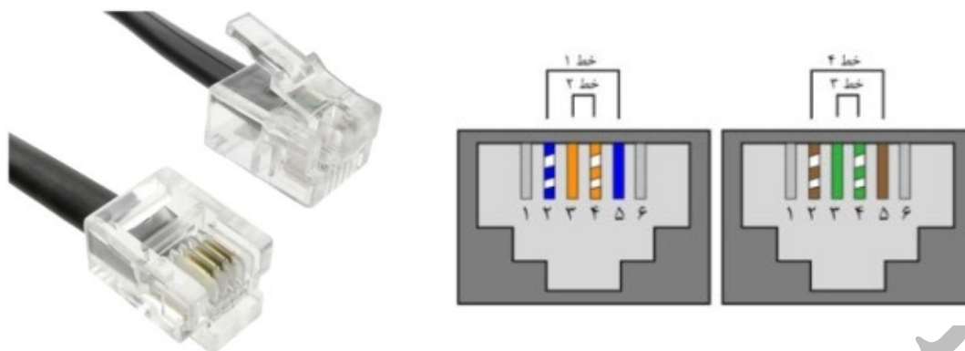
شکل ۱-۳- فیش تلفن RJ11
