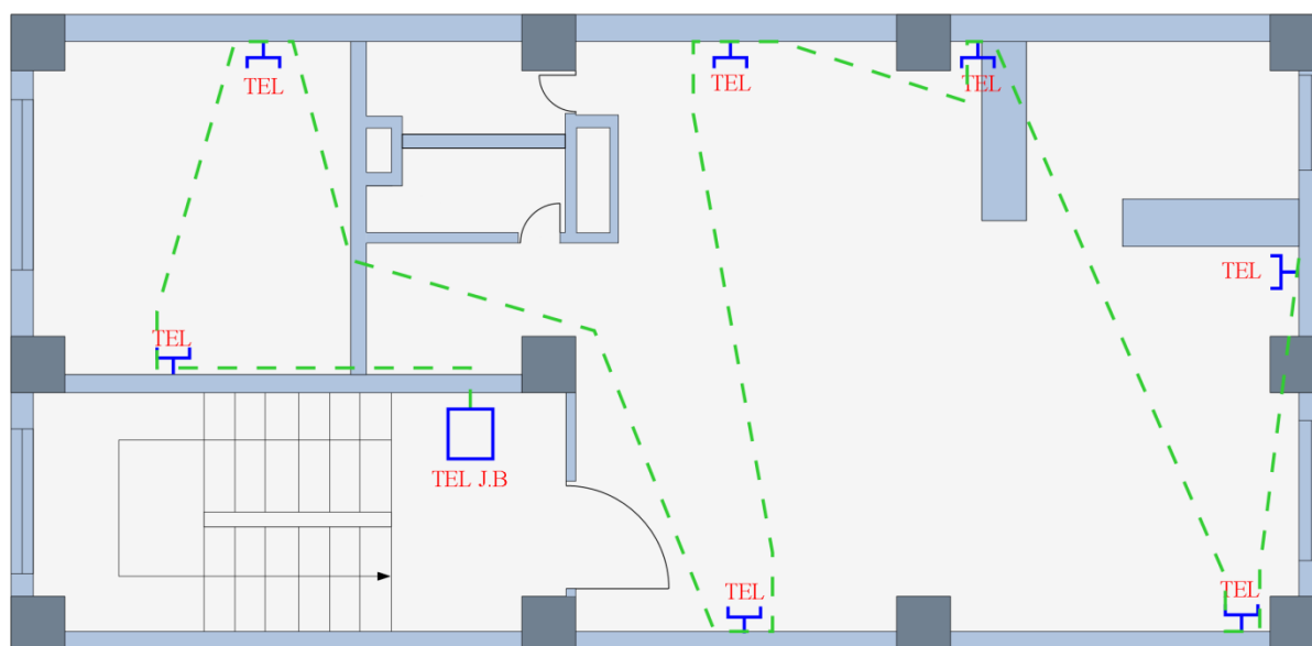
شکل ۱-۱۰- نقشه سیم‌کشی پریز تلفن
