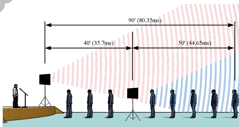
شکل ۷-۲- زمان تاخیر بین دو بلندگو و شنونده
