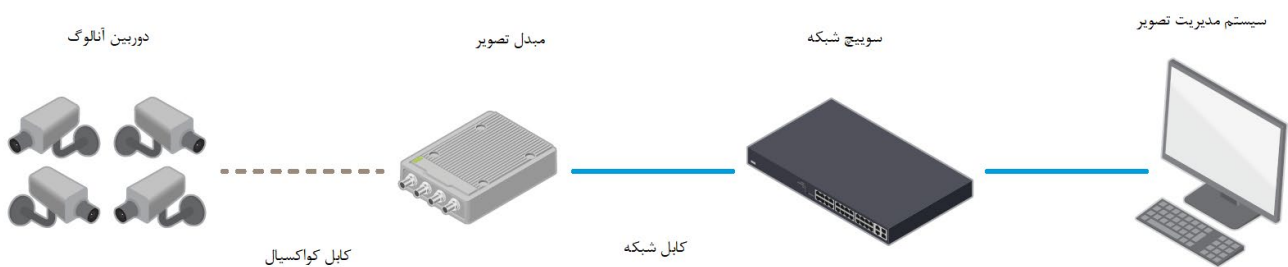
شکل ۳-۲۶- یک نمونه استفاده از مبدل جهت تبدیل ویدیوی آنالوگ دریافتی به ویدیوی دیجیتال
