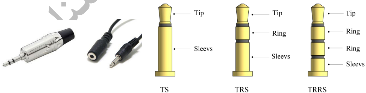
شکل ۷-۱۴۸- دو نمونه جک مادگی و فیش نری ۳٫۵mm
