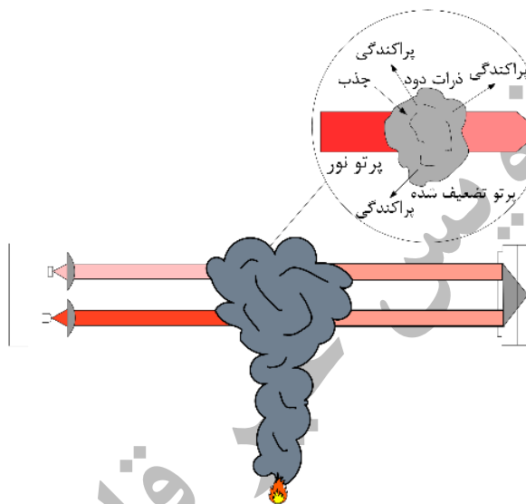
شکل ۴-۱۱- عملکرد دتکتور دودی خطی نوع منعکس کننده
