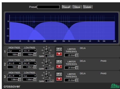
شکل ۷-۶۱- نمونه نرم افزار کنترل کراس اور دیجیتال
