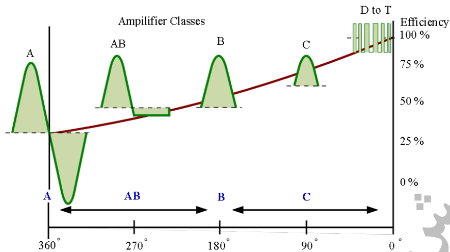
شکل ۷-۸۹- منحنی مقایسه چند کلاس مختلف از تقویت کننده‌ها
