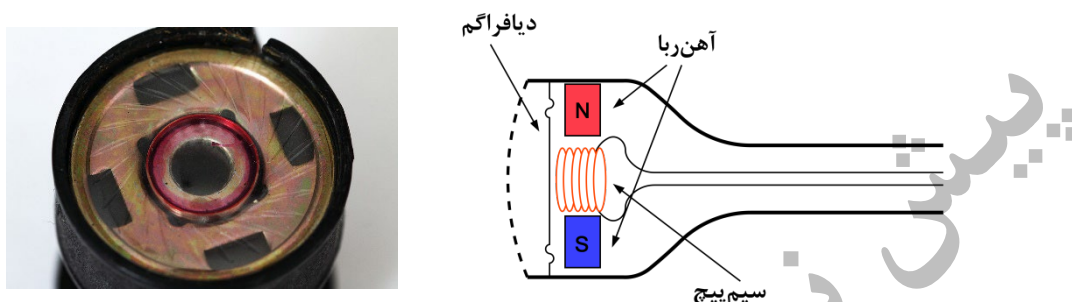
شکل ۷-۲۶- ساختمان داخلی و یک نمونه کپسول میکروفن داینامیک
