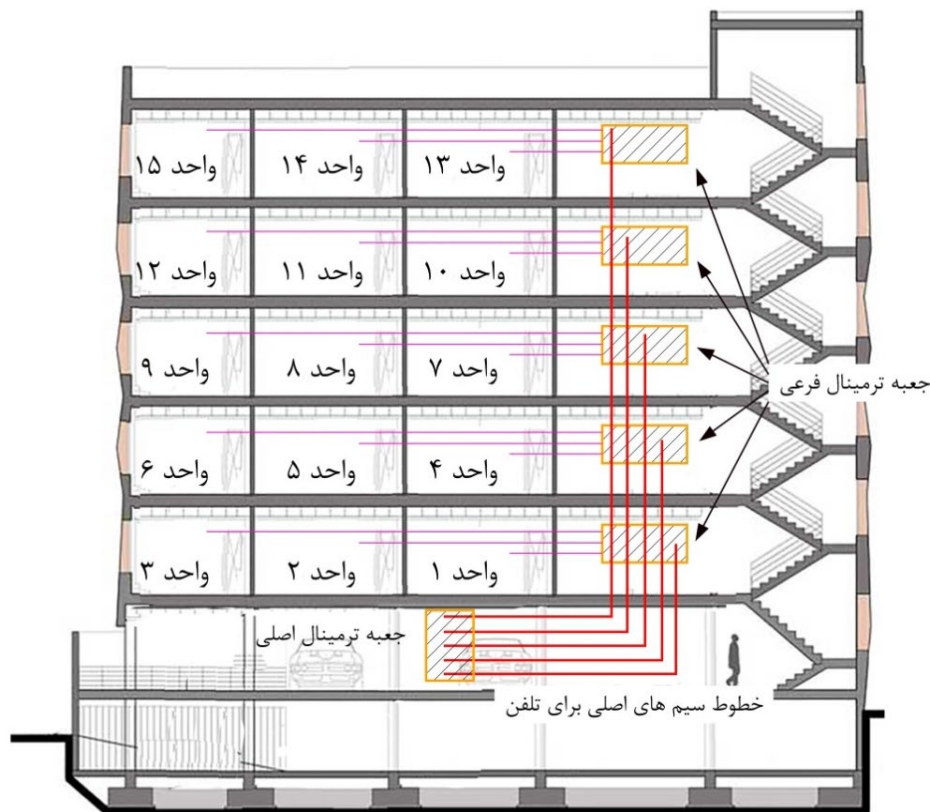
شکل ۱-۱۳- سیم‌کشی تلفن (روش اول)
