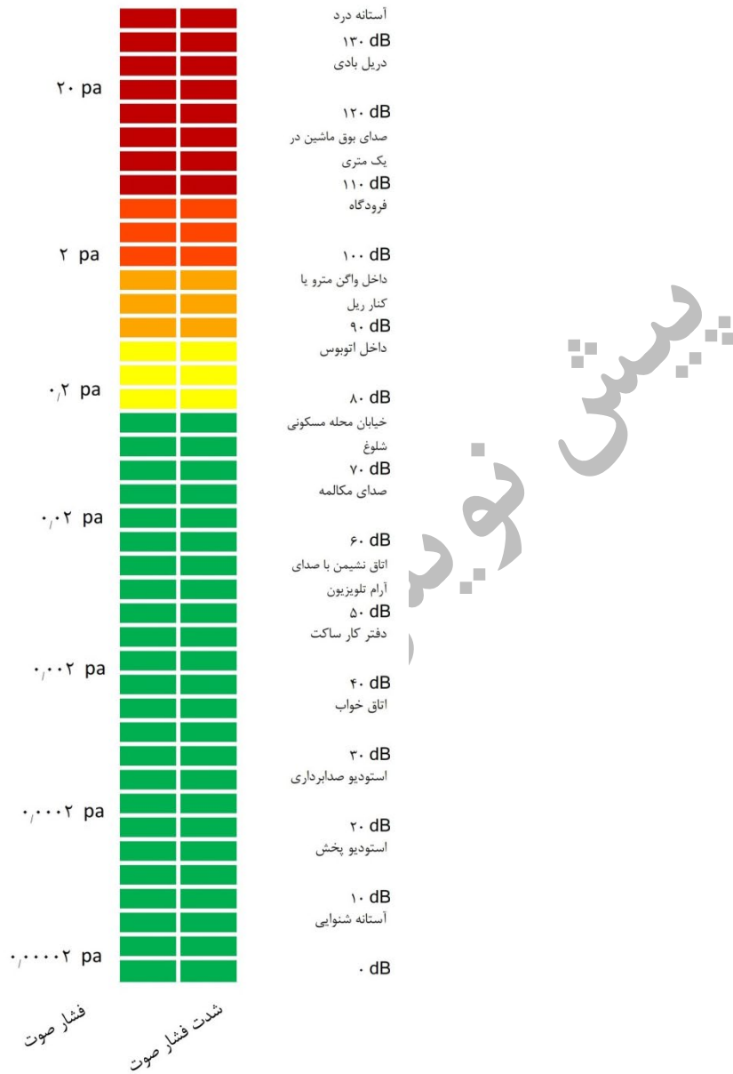
شکل ۷-۵- شدت فشارهای صوت مختلف بر حسب پاسکال و dB
