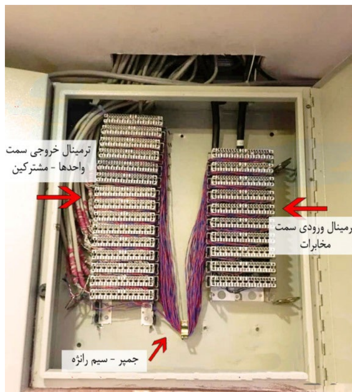
شکل ۱-۱- جعبه ترمینال اصلی تلفن
