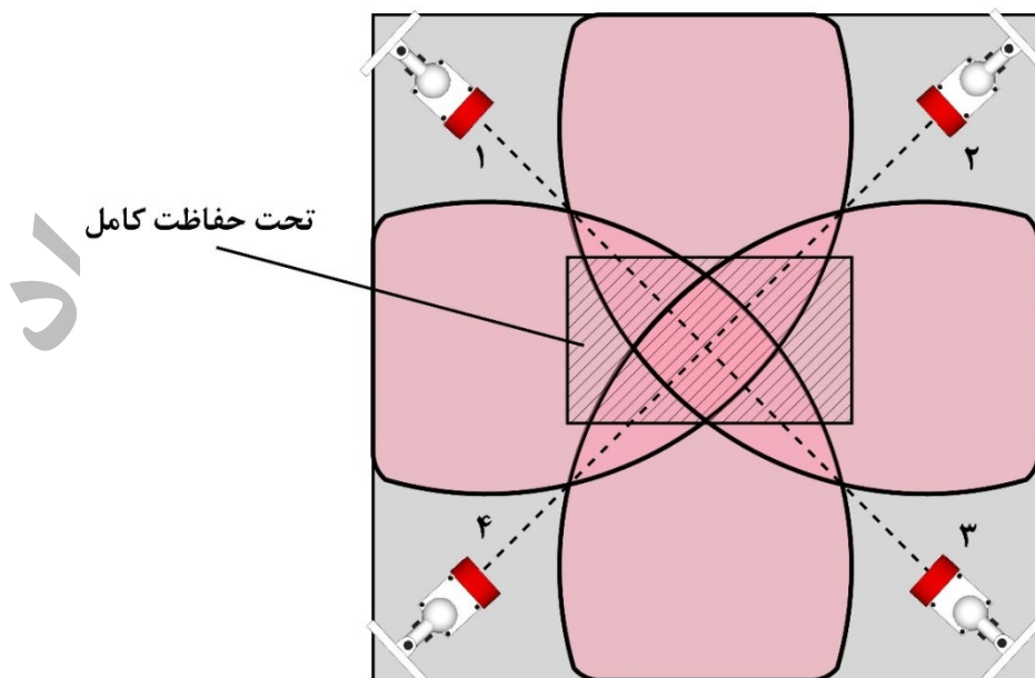
شکل ۴-۶۲- مثالی از جبران کامل اثر سایه
