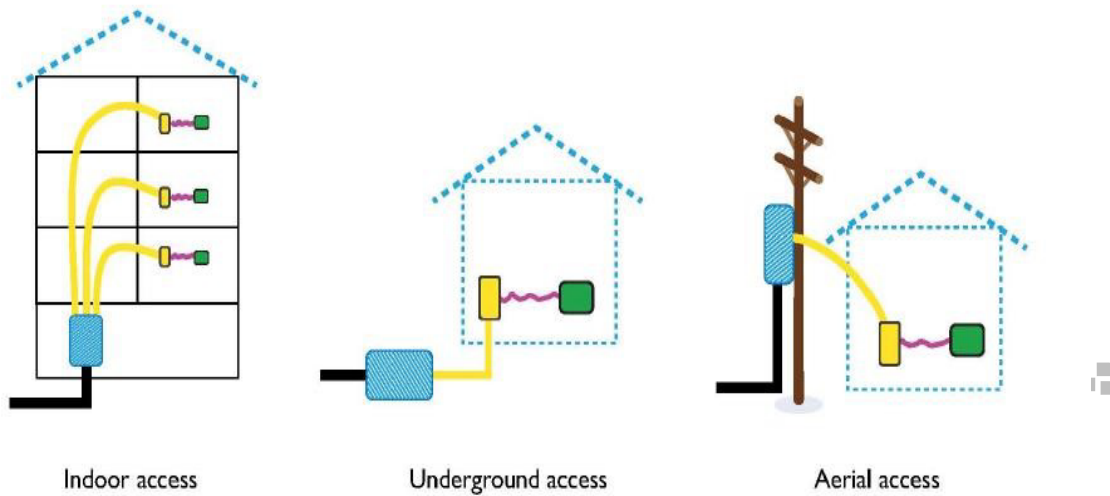
شکل ۱-۱۸- انواع روش‌های ورود به منازل
