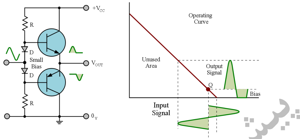
شکل ۷-۹۲- یک نمونه مدار ساده و منحنی نقطه کار و خط بار تقویت کننده کلاس AB
