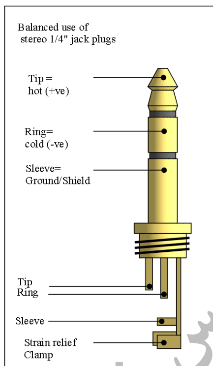
شکل ۷-۱۴۵- نام گذاری و اتصال پایه‌ها در فیش TRS
