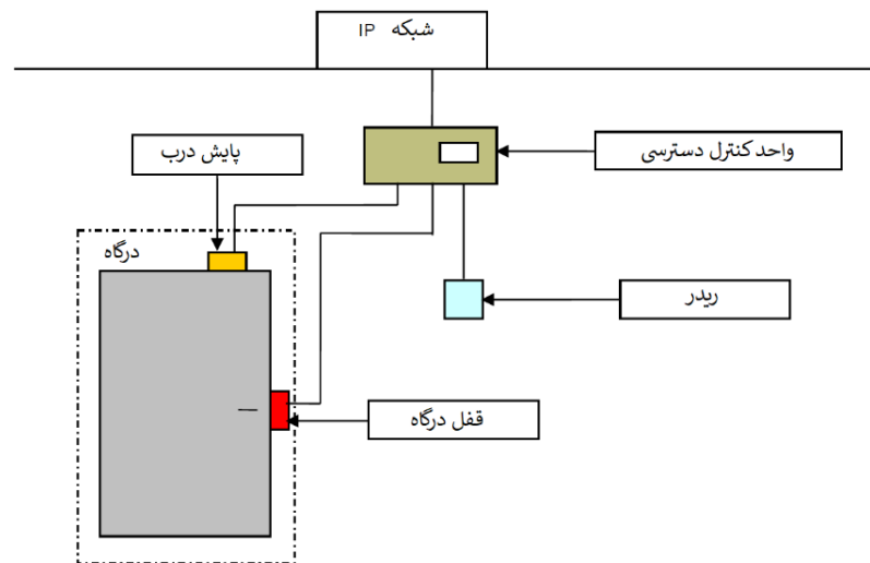
شکل ۳-۲۷- شمای کلی از یک درگاه مجهز به سیستم کنترل دسترسی الکترونیکی تحت شبکه
