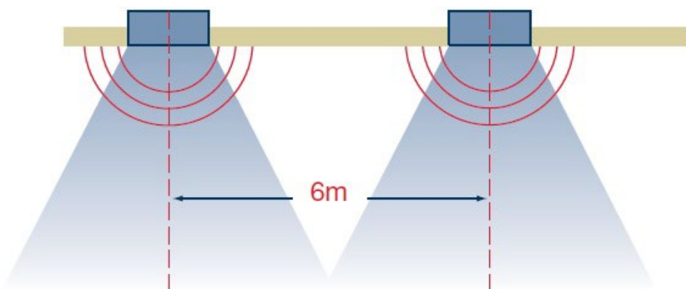
شکل ۵-۵ - فاصله مجاز بین بلندگوهای سقفی
