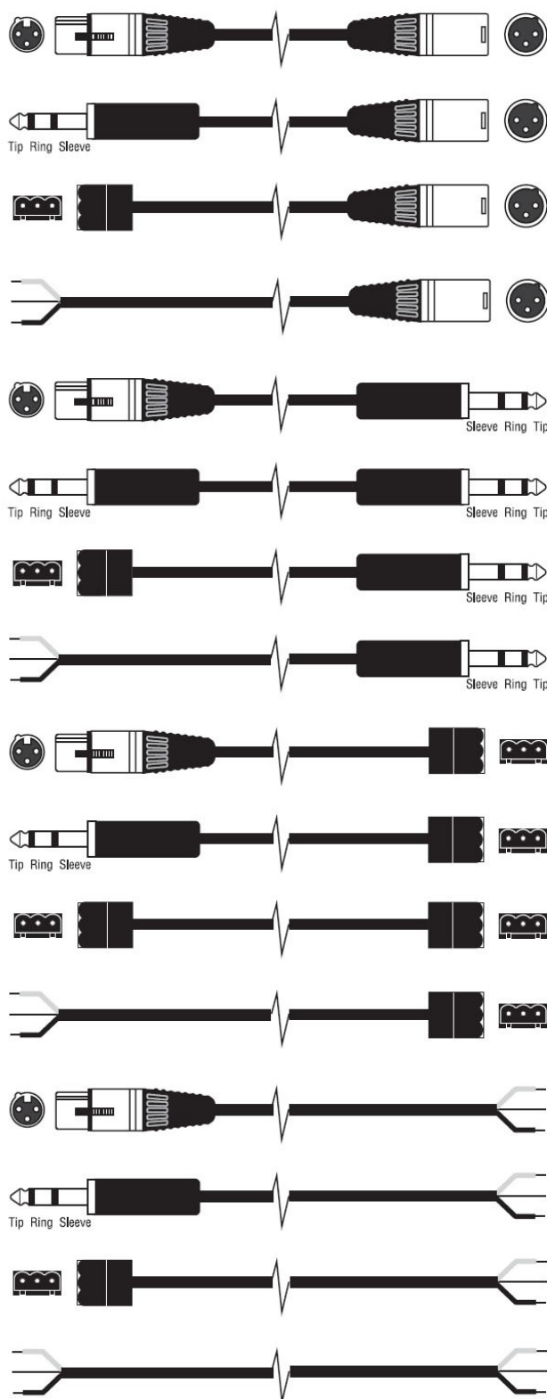
شکل ۷-۱۵۷- نحوه اتصال خروجی سیگنال متوازن به ورودی متوازن با اتصالات مختلف
