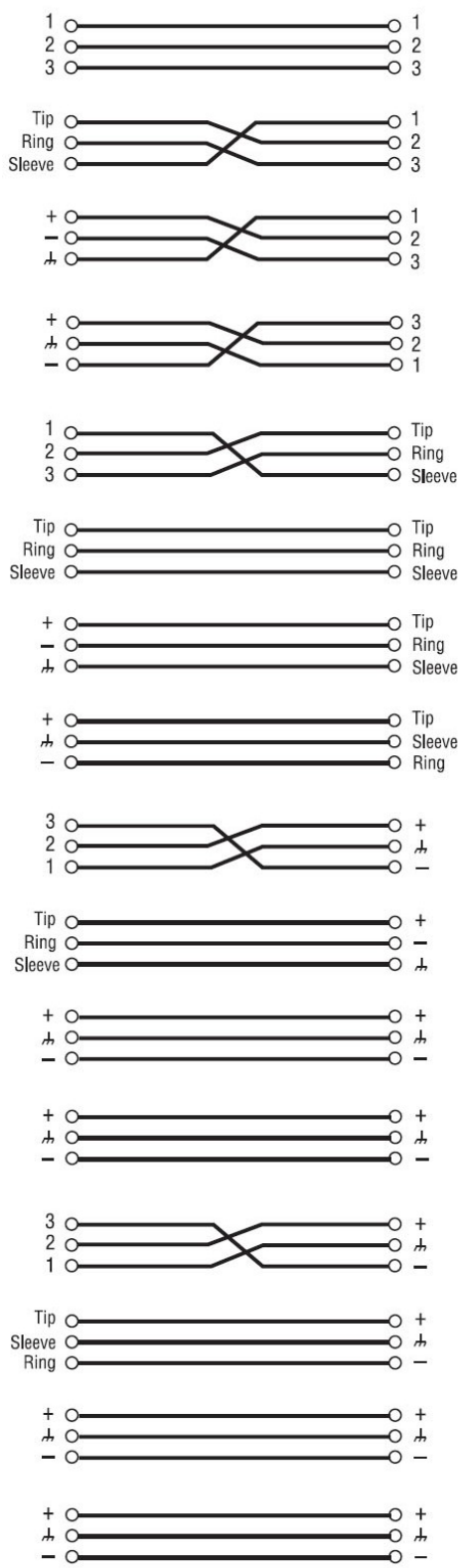
شکل ۷-۱۵۷- نحوه اتصال خروجی سیگنال متوازن به ورودی متوازن با اتصالات مختلف
