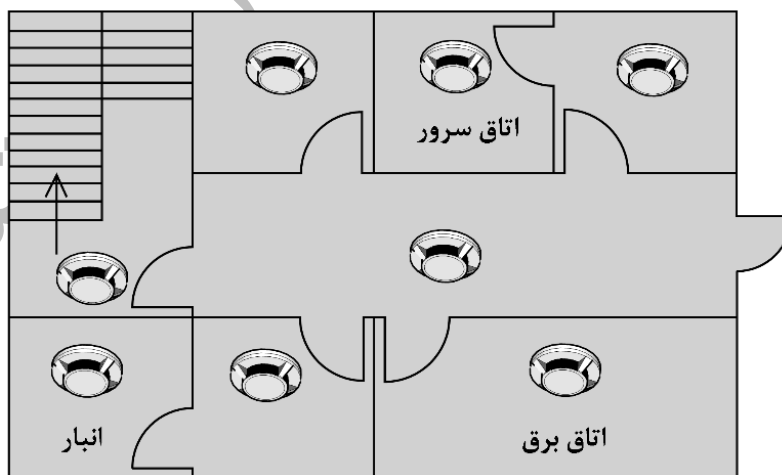
شکل ۴-۱۵- سیستم رسته حفاظت از اموال
