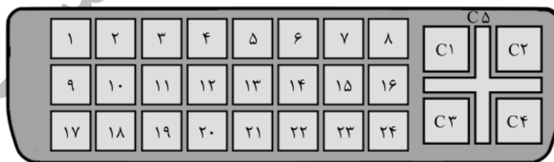
شکل ۸-۲۵- نمای روبروی سوکت مادگی DVI-I
