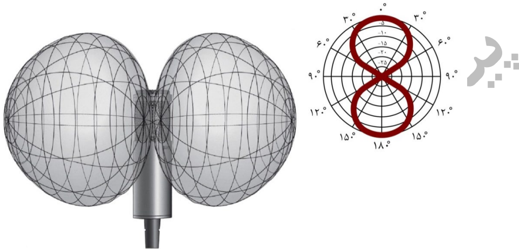
شکل ۷-۲۵- منحنی و بالن الگوی دریافت میکروفن دو جهته یا الگوی ۸
