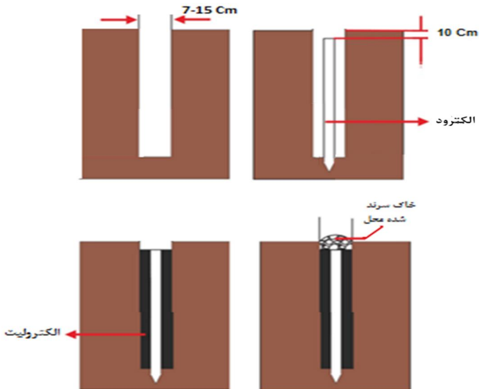
شکل (۱-۲): نحوه استفاده از الکتروولیت اطراف الکترودهای میله‌ای برای موارد خاص (دریچه بازدید برای سادگی در شکل نشان داده نشده است).
